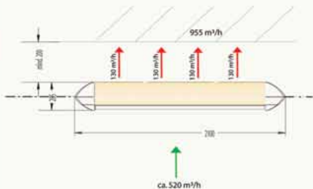
Schemat przepływu powietrza
